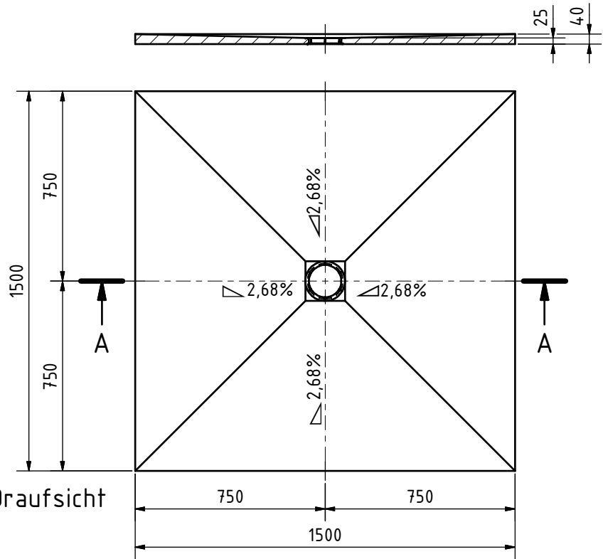
Ansicht A-A
