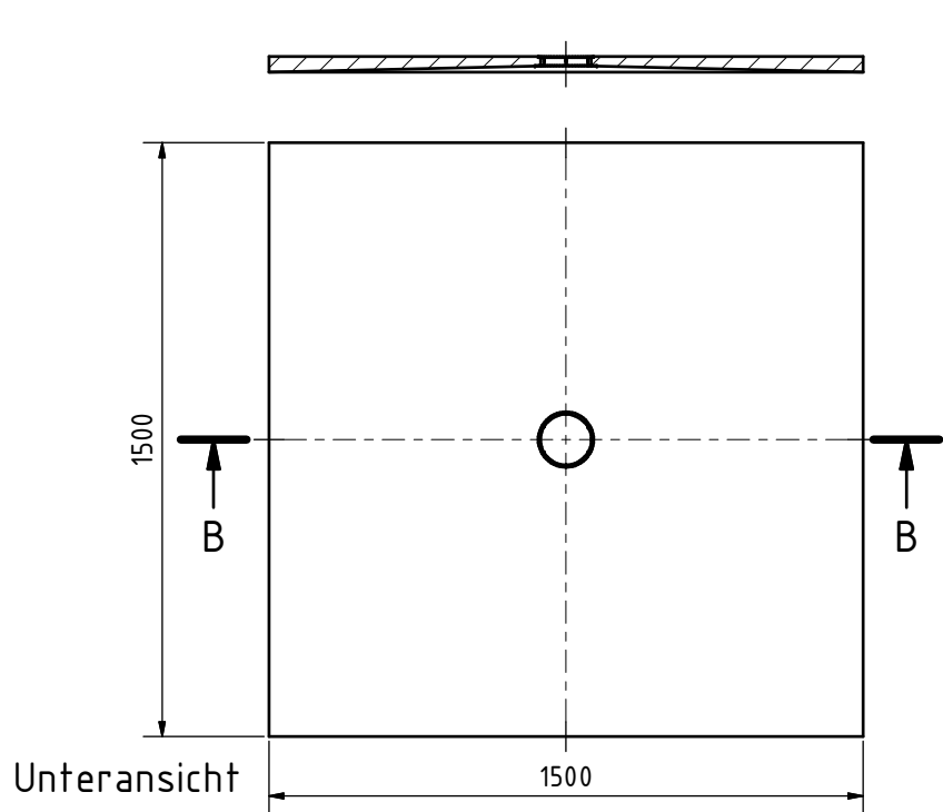
Ansicht B-B
