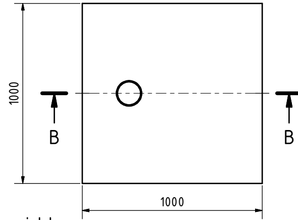
Unteransicht
